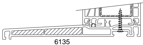
EMBOUT 9F54.1(2 PIECES) POUR 6135
