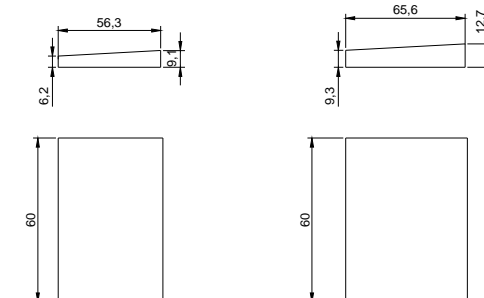
EMBOUT 9F54.1(2 PIECES) POUR 6135
