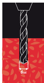
Percer le trou à Ø d_{cut} et profondeur mini h_1
