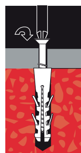
Poser l'objet en réalisant l'expansion de la cheville avec une «vis bois»
